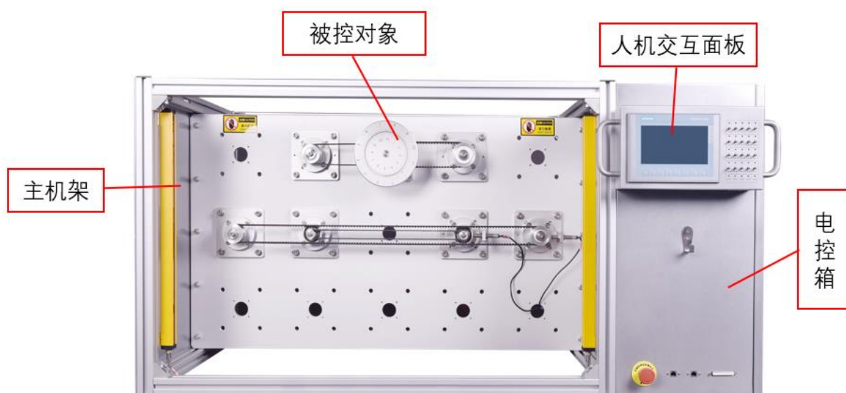
图 1-1 设备示意图
